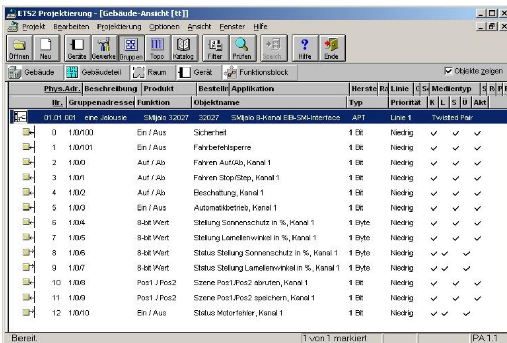
Abb: Kommunikationsobjekte in der ETS (ein Kanal, Jalousie, mit Automatik)
